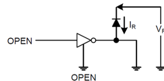
6. I_R
