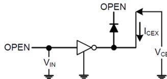
1. I_{CEX}
